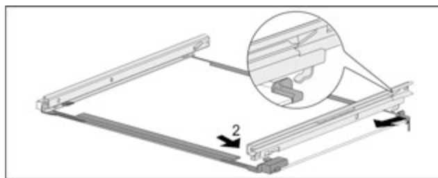
Fig. 149 Скляна пластина з рейками
